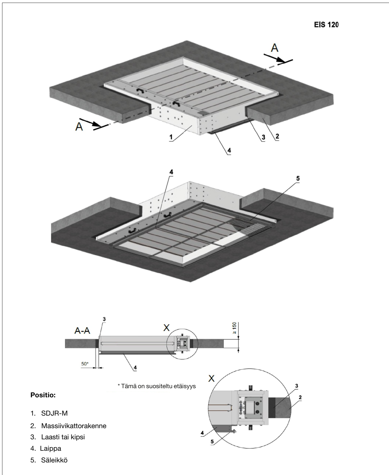
Kuva 31 Kiviaineinen katto/lattiarakenne
