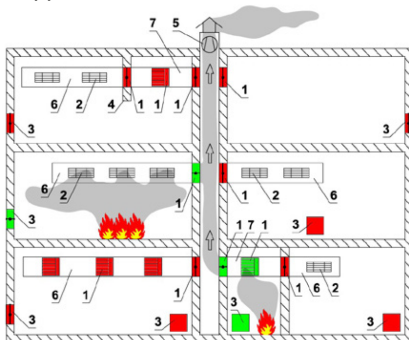
Kuva 1 Esimerkki koneellisen savunhallintajärjestelmän osista
