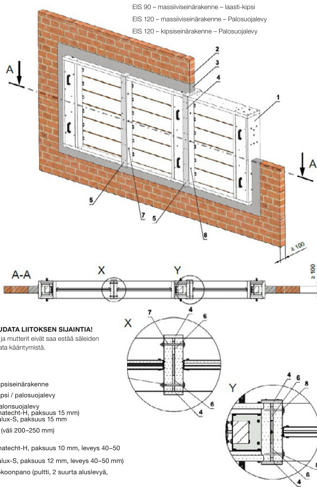
Kuva 29 Kolme savunhallintapeltiä vierekkäin – massiivi-/kipsilevyseinärakenne – laasti tai kipsi / palosuojalevy
