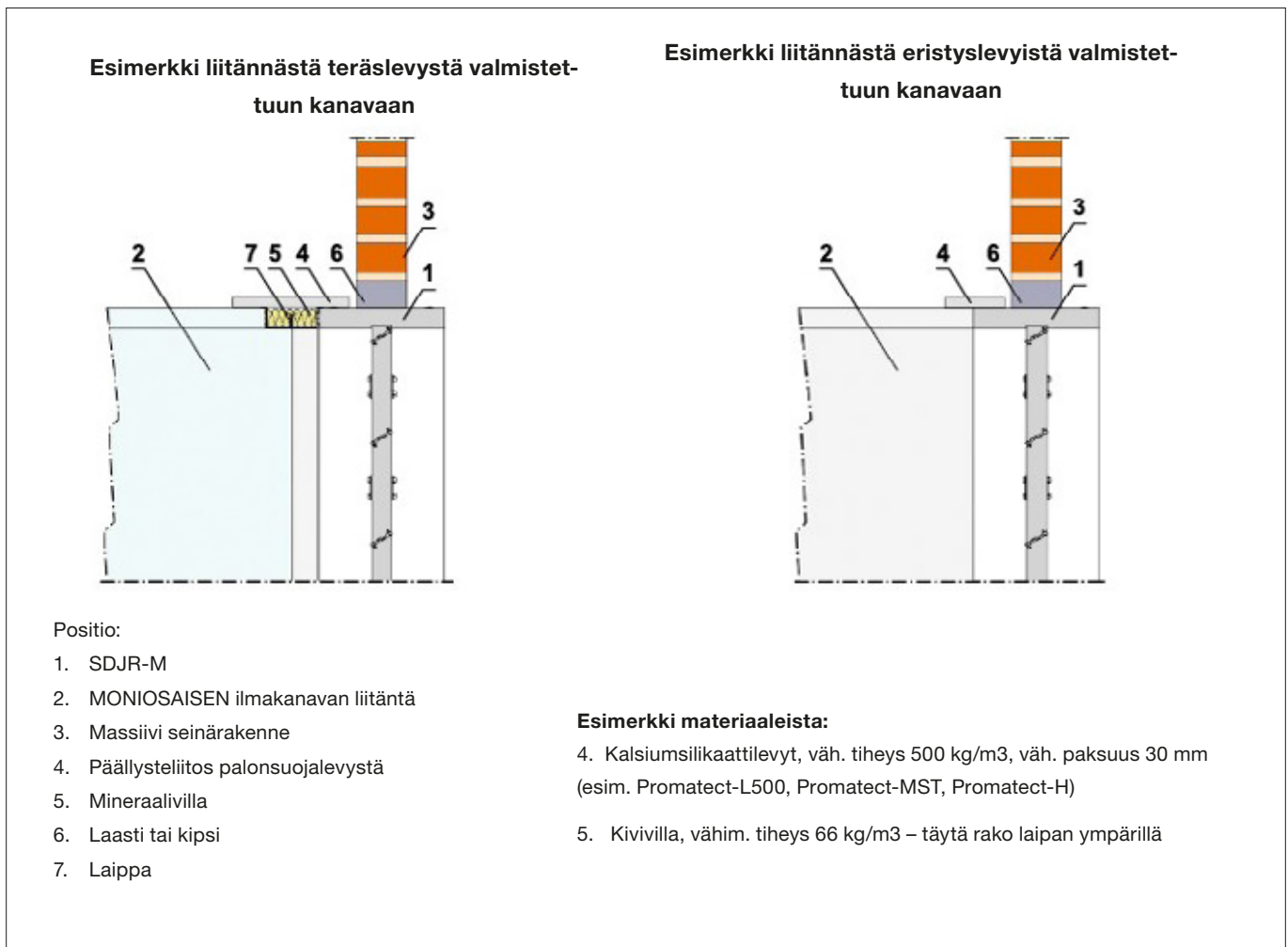
Kuva 36 Esimerkki liitännästä vaakasuoraan kanavaan
