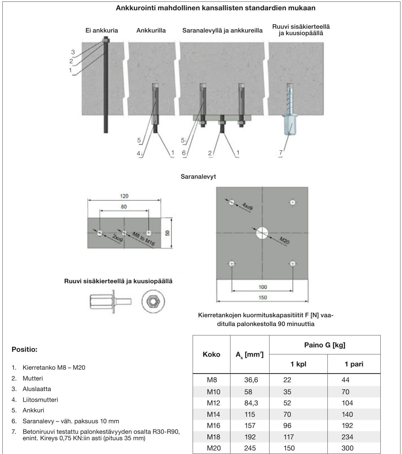
Kuva 31 Kiinnitys kattorakenteeseen
