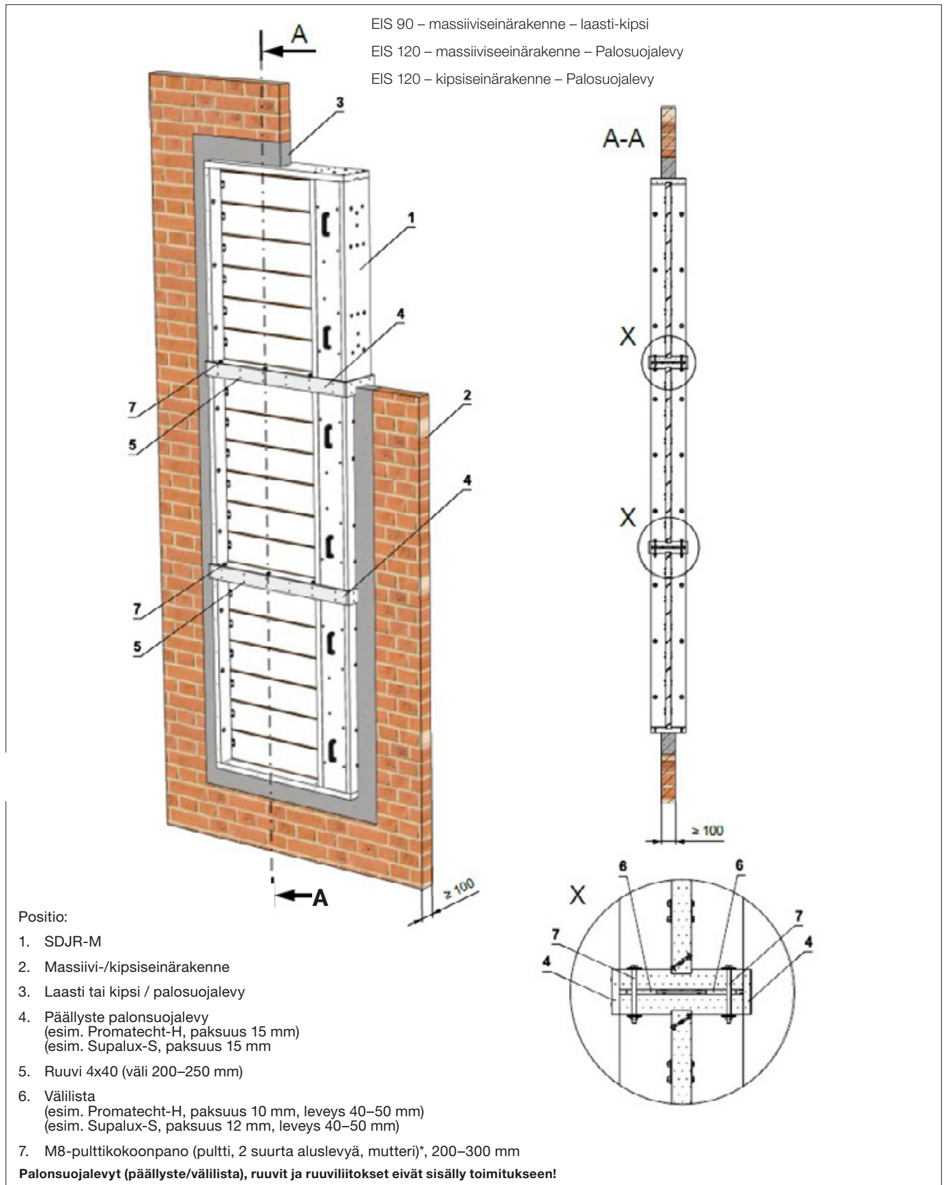
Kuva 30 Kolme savunhallintapeltiä päällekkäin – massiivi-/kipsilevyseinärakenne – laasti tai kipsi / palosuojalevy
