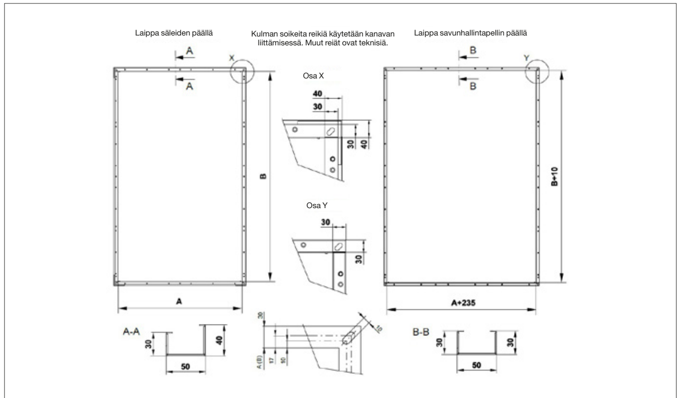
Kuva 17 Laippa (2 tyyppiä)
