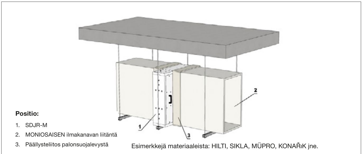
Kuva 35 Esimerkki savunhallintapellin asennuksesta ja ripustuksesta vaakasuoraan kanavaan
