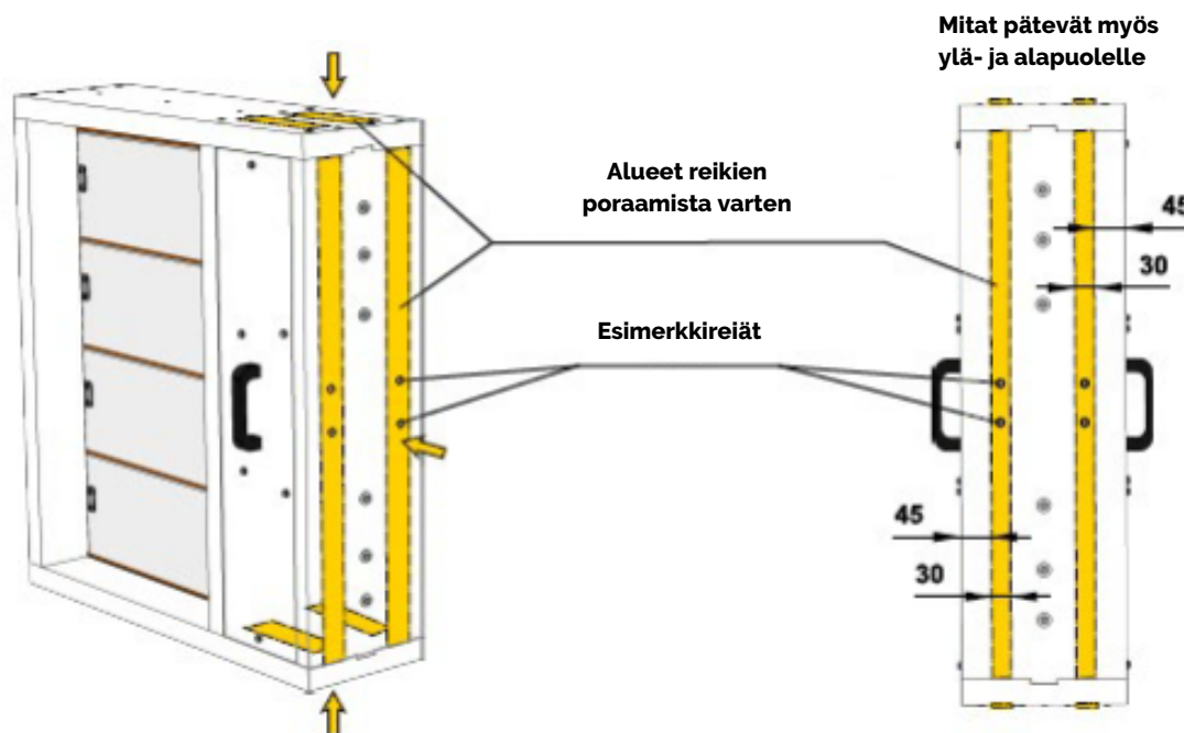
Kuva 37 Esimerkki reikien sijainnista kotelon seinässä ilman valmiita reikiä
