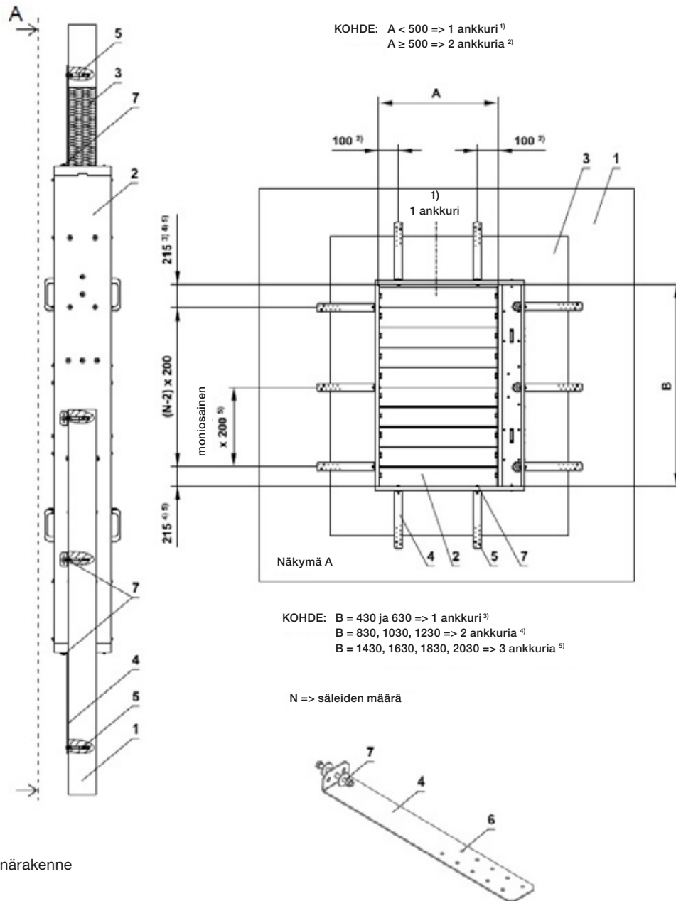
Kuva 32 SDJR-M:n kiinnittäminen massiiviseinärakenteeseen Weichschott/Palosuojalevy -järjestelmällä
