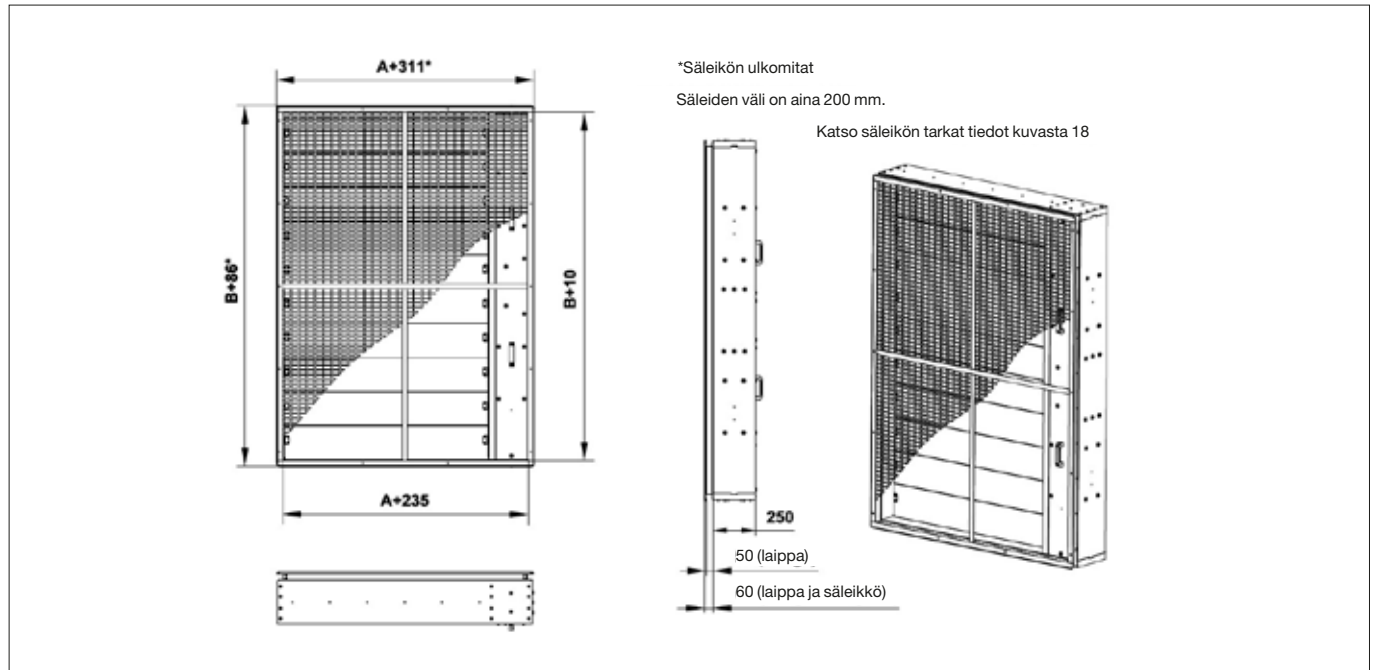
Kuva 16 Laippa ja säleikkö kehyksen päällä
