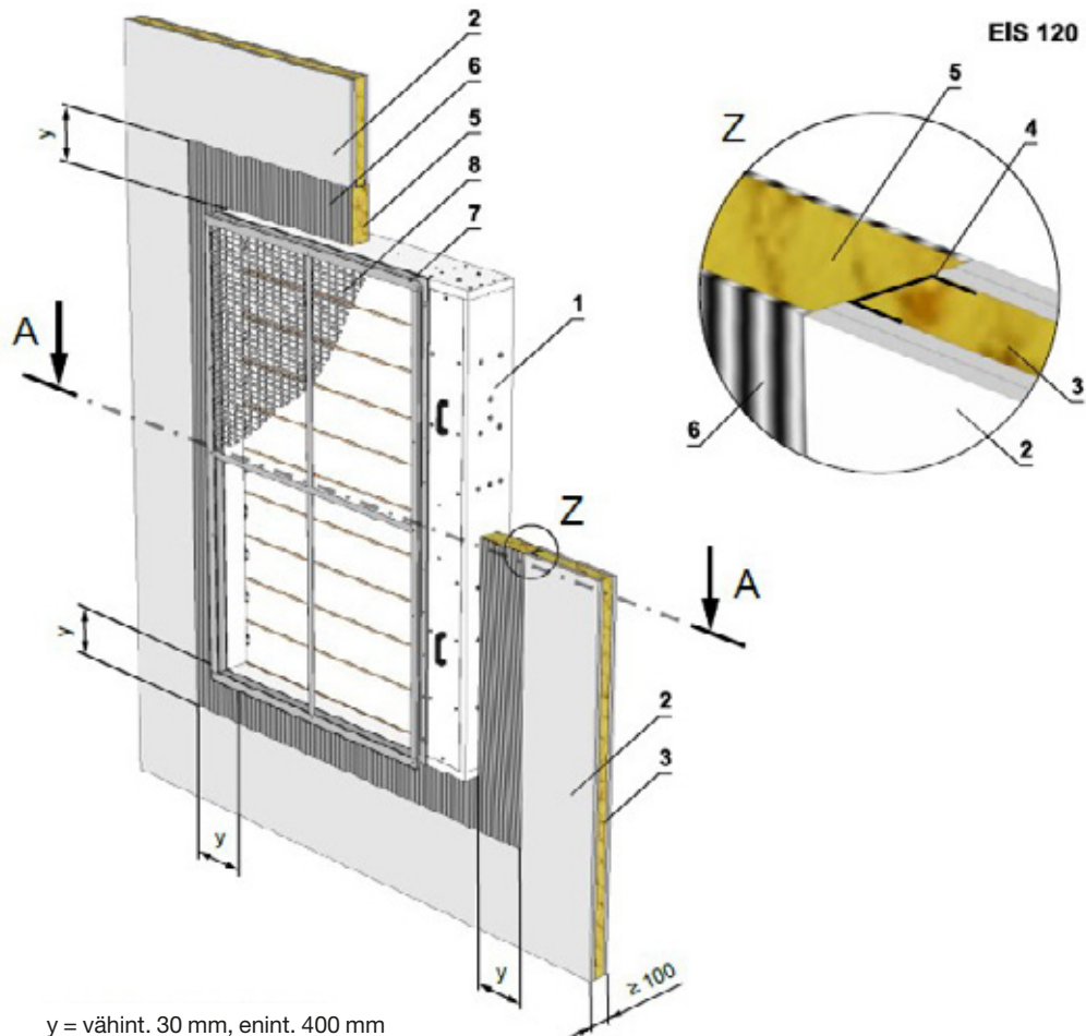
Kuva 25 Kipsilevyseinä/-kuilu rakenne – palosuojalevy
