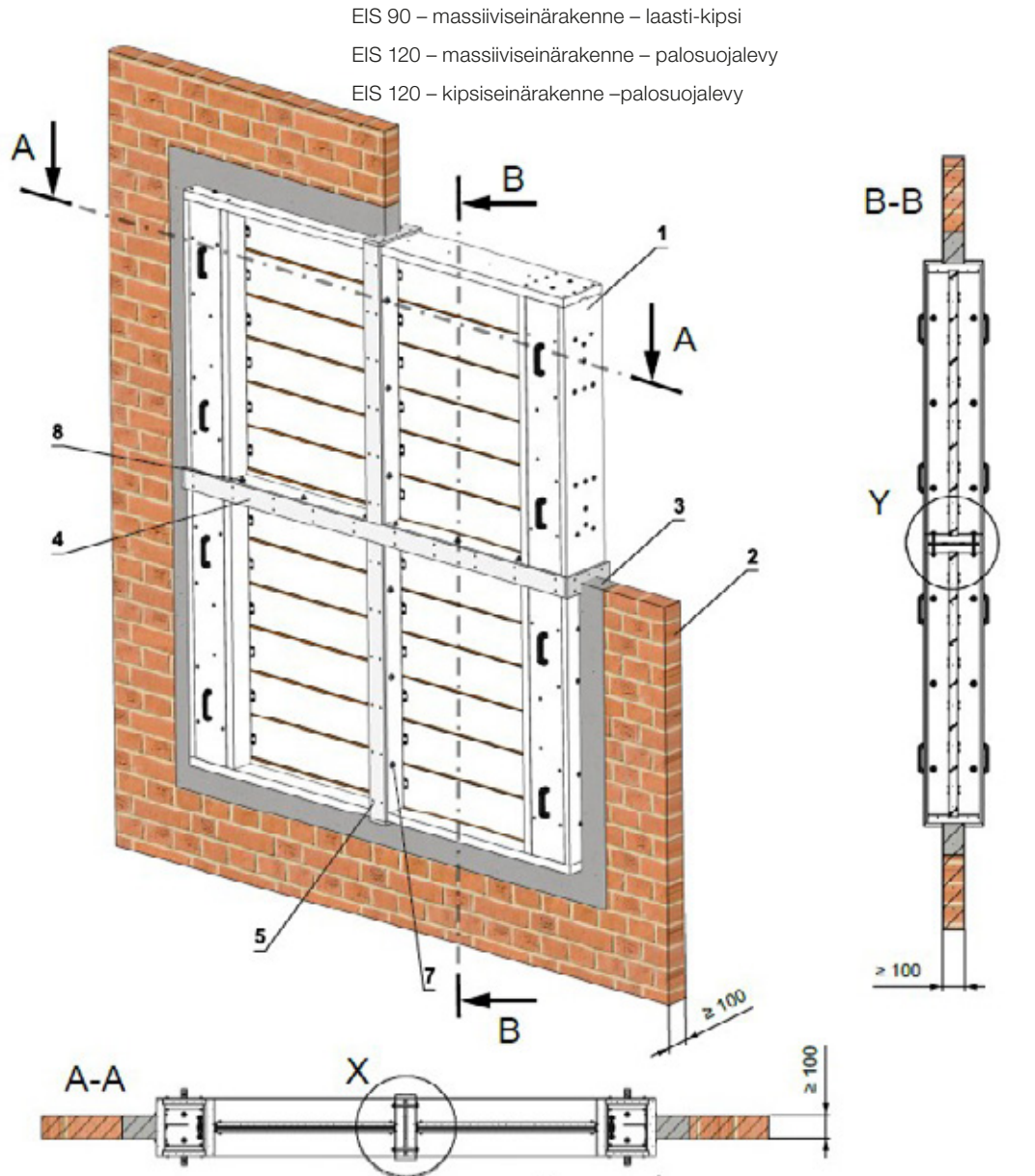
Kuva 28 Neljä savunhallintapeltiä – massiivi-/kipsilevyseinärakenne – laasti tai kipsi / palosuojalevy
