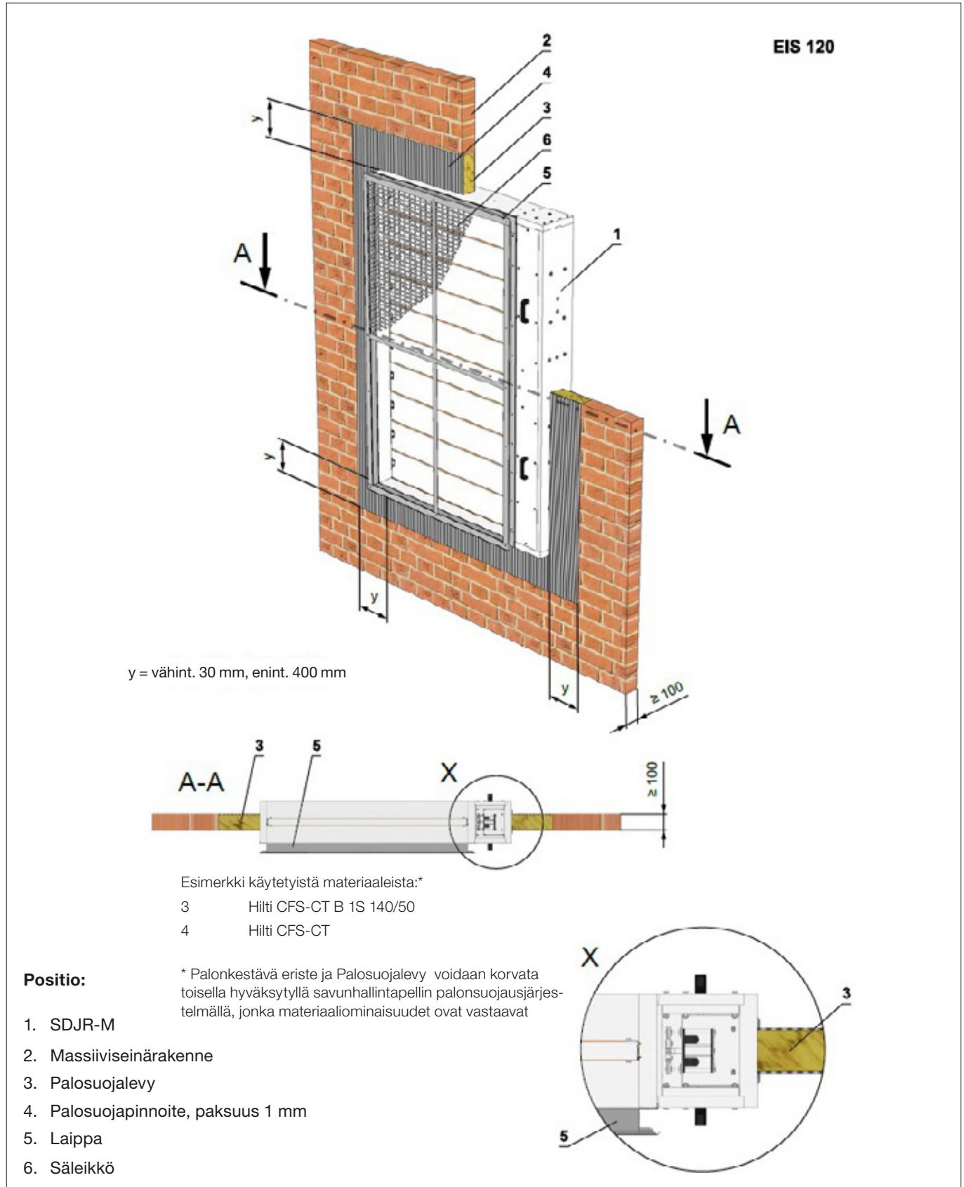
Kuva 24 Massiiviseinä/-kultu – palosuojalevy
