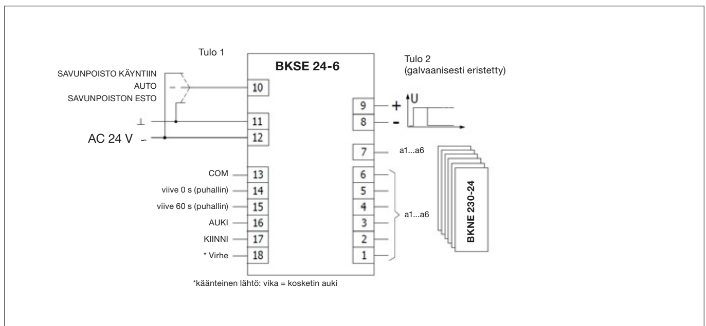
Kuva 13 Tiedonsiirto- ja ohjauslaitteet BKSE 24-6
