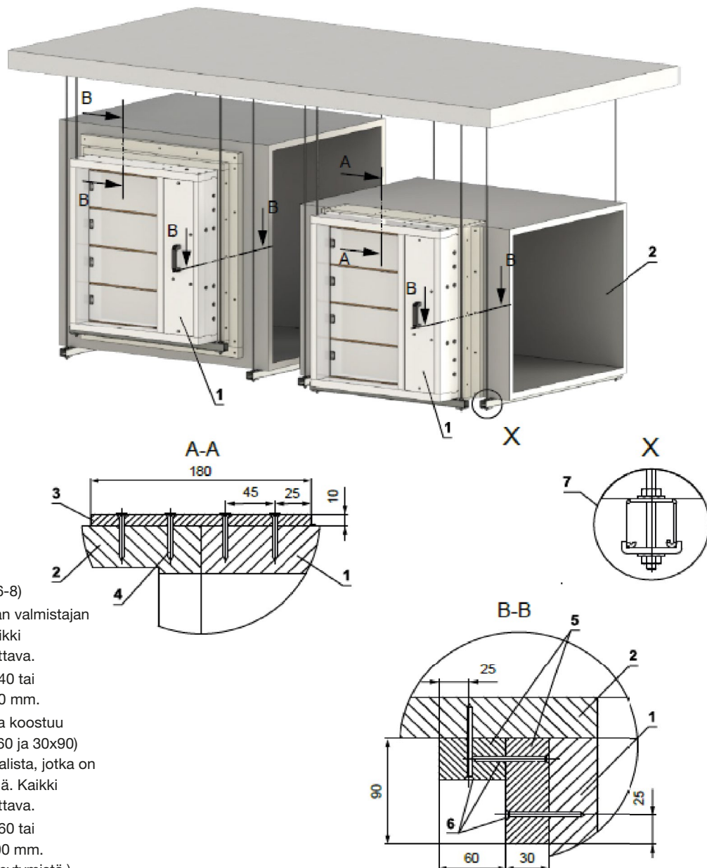
Kuva 34 Esimerkki savunhallintapellin asennuksesta ja ripustuksesta vaakasuoraan kanavaan
