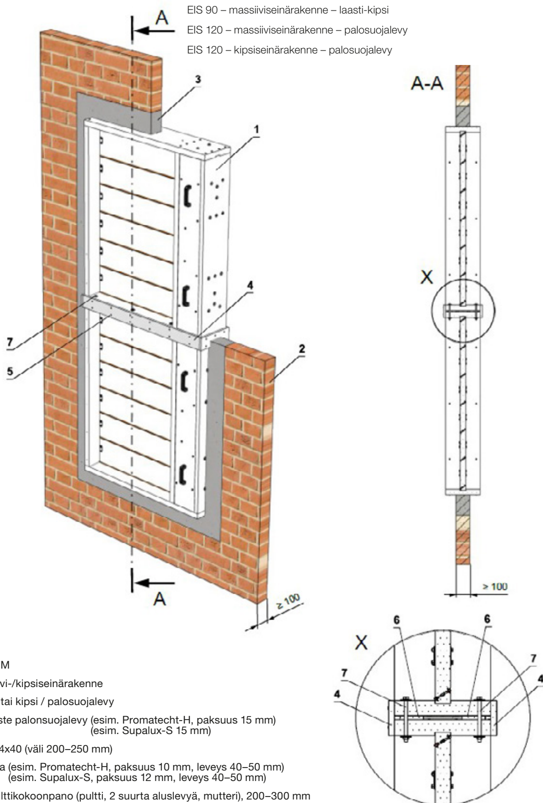
Kuva 27 Kaksi savunhallintapeltiä päällekkäin – massiivi-/kipsilevyseinärakenne – laasti tai kipsi / palosuojalevy
