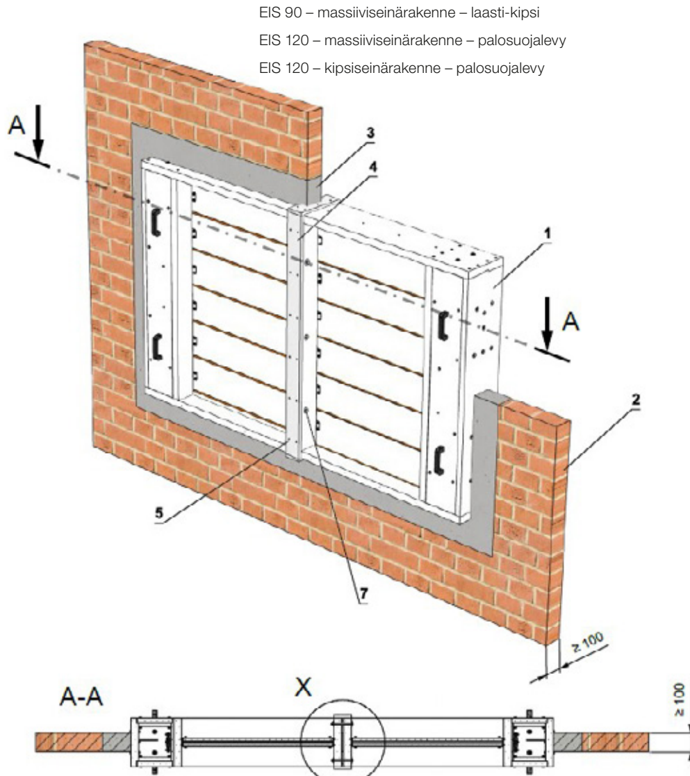
Kuva 26 Kaksi savunhallintapeltiä vierekkäin – massiivi-/kipsilevyseinärakenne – laasti tai kipsi / palosuojalevy
