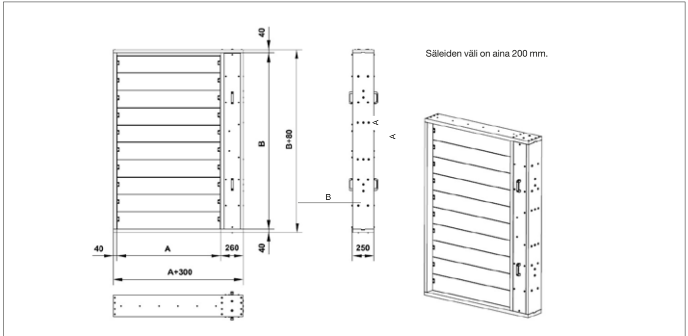
Kuva 14 Ilman laippoja
