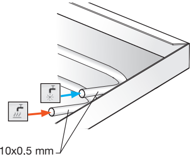
C7: Liitântätyyppi 7: 15-asteen kulma
