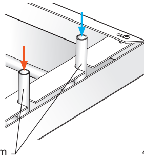
C2: Liitântätyyppi 2: pystysuora
