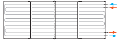
C7: Liitântätyyppi 7: 15-asteen kulma
