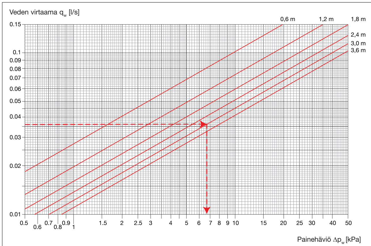
Kaavio 4. Atrium Plana 60, painehäviö 60°C:ssä. Painehäviö muussa kuin 60°C:n lämpötilassa saadaan kertomalla painehäviö painehäviökertoimella (katso kaavio 5).
