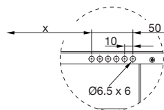
Kannattimien asennustapa (4 kpl jos L_{nom} < 2,4 m ja 6 kpl jos L_{nom} \geq 2,4 m)
