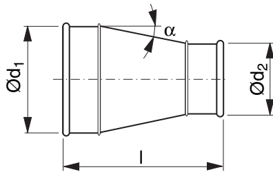
Tuotekuvas Pitkä keskeismuuntoyhde noin 18° kulmalla.
